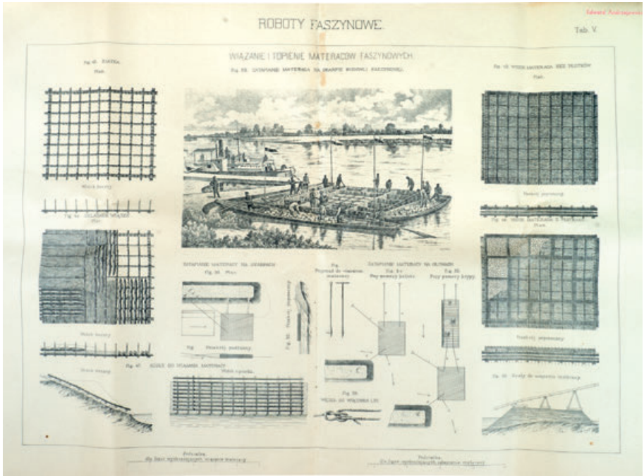
661. J. Ćwikiel. Budowle wodne na Wiśle. 1925.
